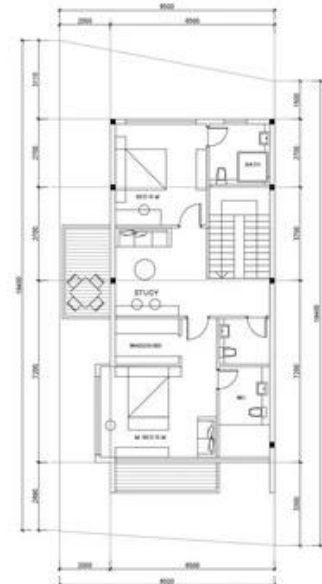
MẶT BẰNG TẦNG 3
