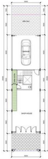
MẶT BẰNG TẦNG 1
