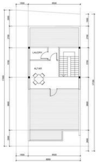
MẶT BẰNG TẦNG THƯỢNG
