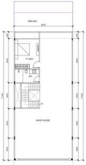
MẶT BẰNG TẦNG 2 CONSTRUCTION AREA: 134.3 m 2
