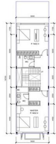
MẶT BẰNG TẦNG 4
