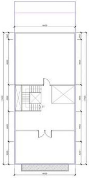
MẶT BẰNG SÂN THƯỢNG CONSTRUCTION AREA: 127.3 m 2 BALCONY AREA: 5.5 m 2
