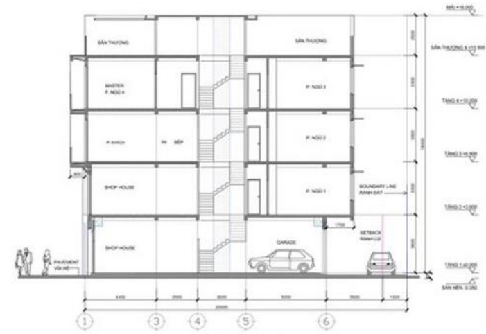
MẶT CẮT ĐỌC
