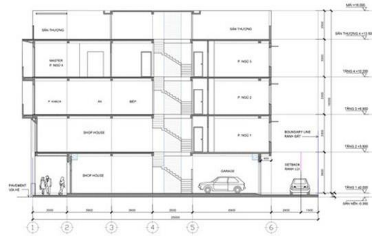
MẶT CẮT DỌC
