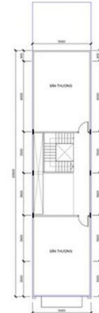
MẶT BẰNG SÂN THƯỢNG
