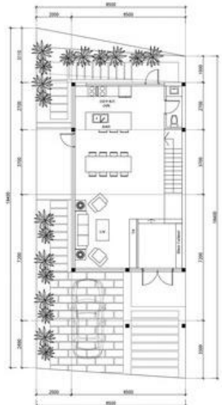
MẶT BẰNG TẦNG 1
