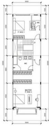
MẶT BẰNG TẦNG 2
