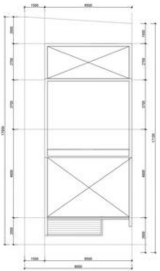
MẶT BẰNG MÁI
