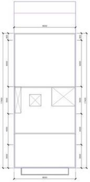
MẶT BẰNG MÁI
