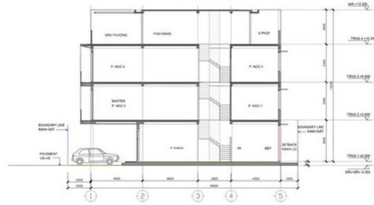
MẶT CẮT DỌC
