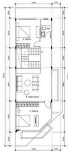
MẶT BẰNG TẦNG 3
