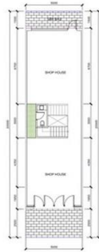
MẶT BẰNG TẦNG 1
