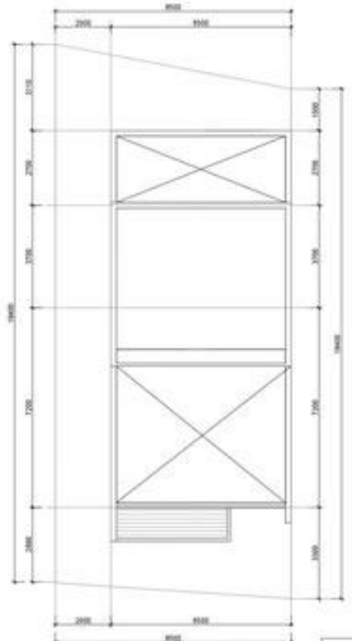
MẶT BẰNG MÁI
