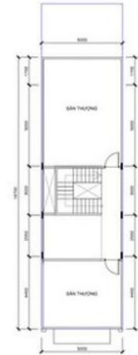
MẶT BẰNG TẦNG THƯỢNG
