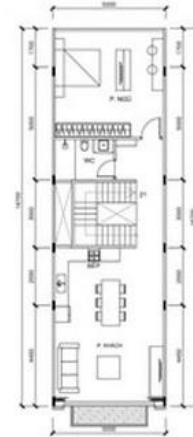
MẶT BẰNG TẦNG 3
