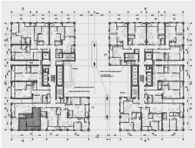
MẪU CĂN HỘ 1 PHÒNG NGỦ DIỆN TÍCH : 59,3 m 2 (Kích thước thực tế xác định theo bản vẽ hoàn công)
