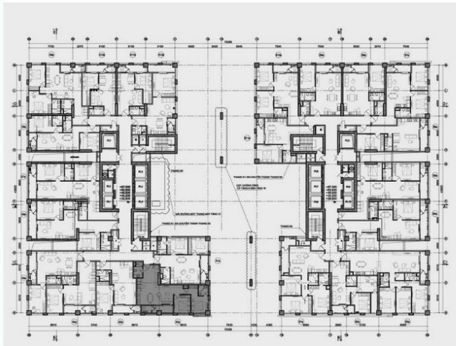
MẪU CĂN HỘ 2 PHÒNG NGỦ DIỆN TÍCH : 75,9 m 2 (Kích thước thực tế xác định theo bản vẽ hoàn công)
