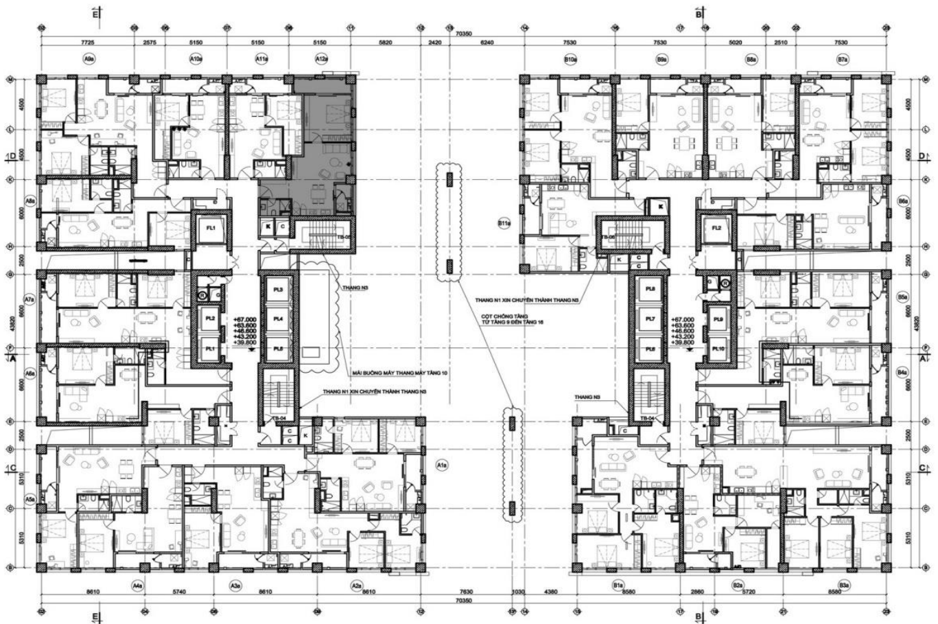
MẪU CĂN HỘ 1 PHÒNG NGỦ DIỆN TÍCH : 62,8 m 2 (Kích thước thực tế xác định theo bản vẽ hoàn công)
