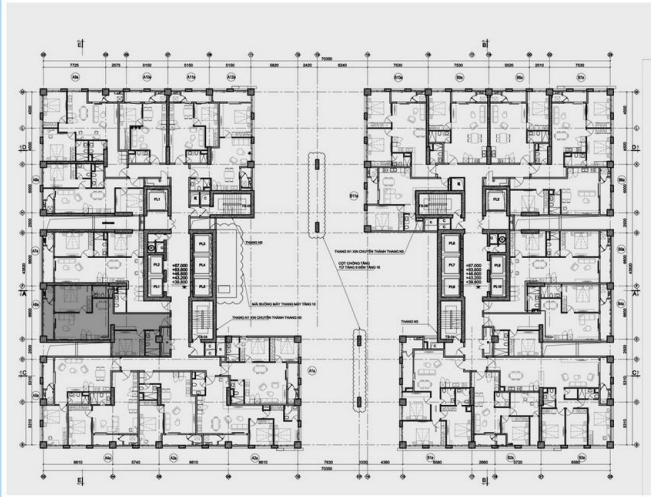
MẪU CĂN HỘ 2 PHÒNG NGỦ DIỆN TÍCH : 90 m 2 (Kích thước thực tế xác định theo bản vẽ hoàn công)
