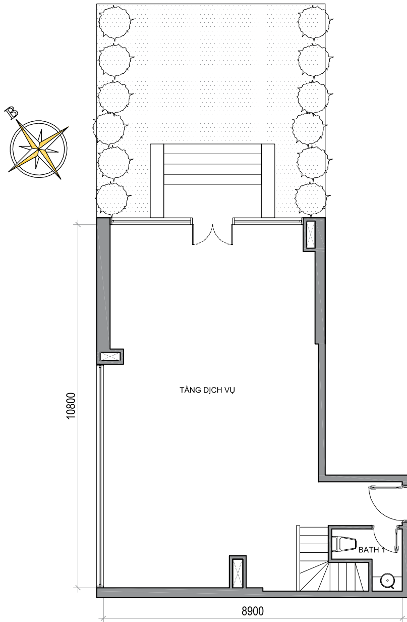
TẦNG TRỆT
