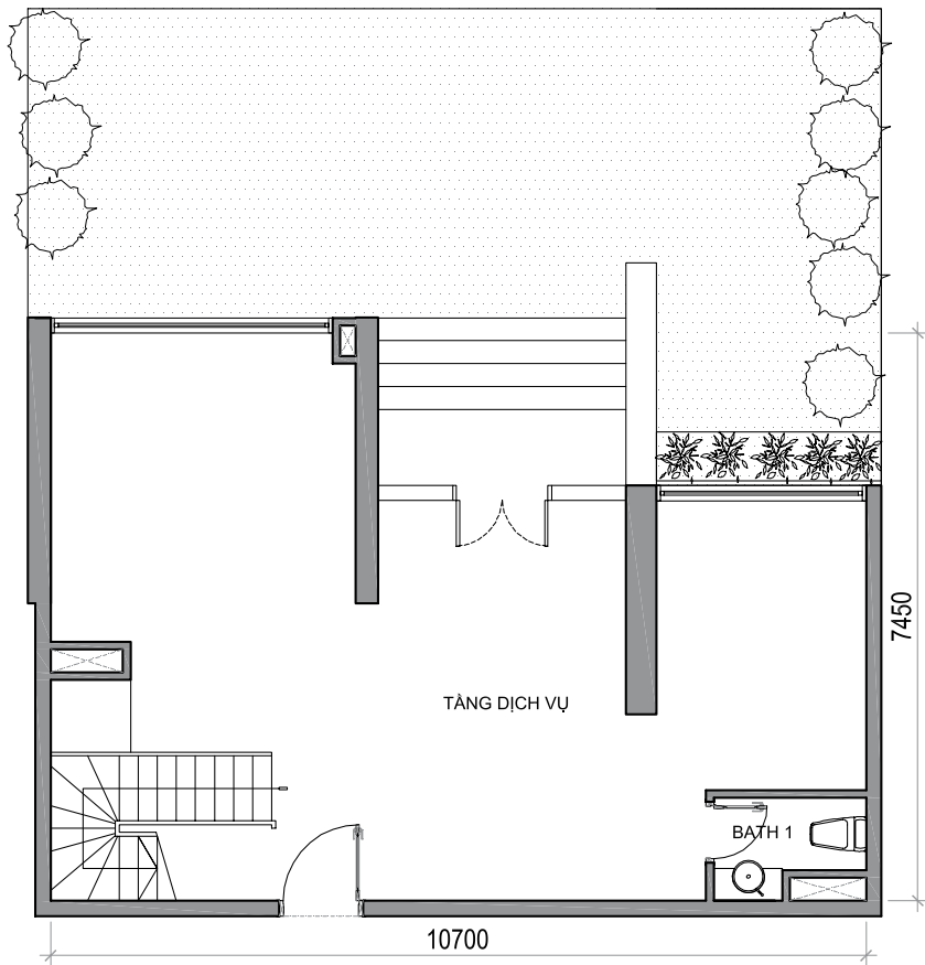
TẦNG TRỆT
