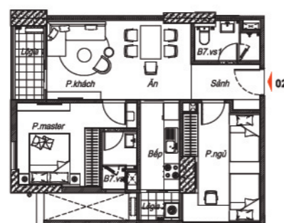
Tầng 7 - 10 & 16 - 20
