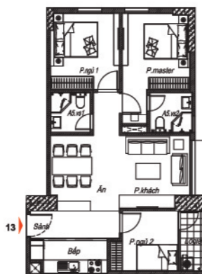
Tầng 7 - 10 & 16 - 20
