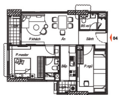
Tầng 11 - 15 & 21 - 26
