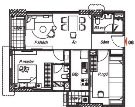
Tầng 11 - 15 & 21 - 26
