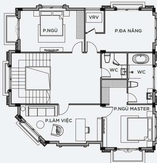
MẶT BẰNG TẦNG 3
