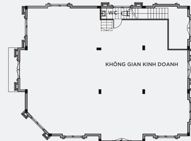
MẶT BẰNG TẦNG 1
