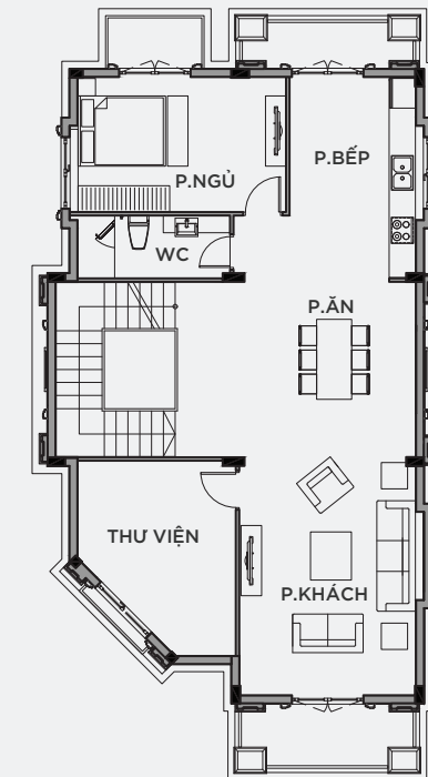
MẶT BẰNG TẦNG 2
