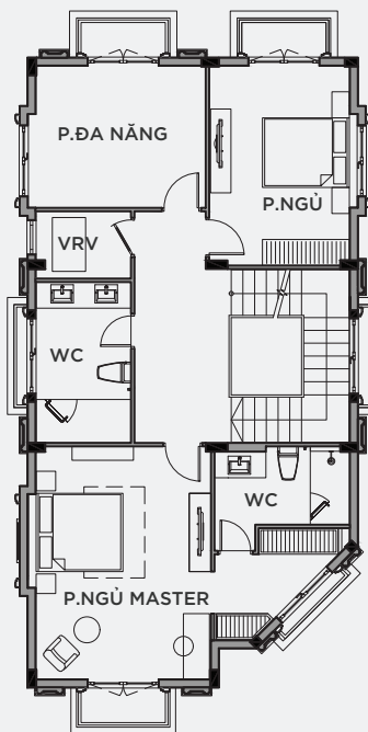
MẶT BẰNG TẦNG 3
