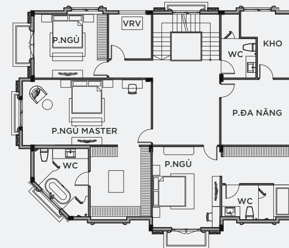
MẶT BẰNG TẦNG 3
