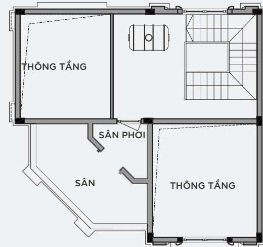
MẶT BẰNG ÁP MÁI
