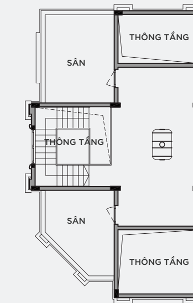
MẶT BẰNG ÁP MÁI
