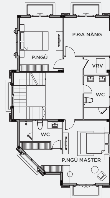
MẶT BẰNG TẦNG 3
