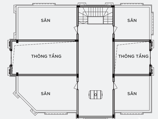
MẶT BẰNG ÁP MÁI
