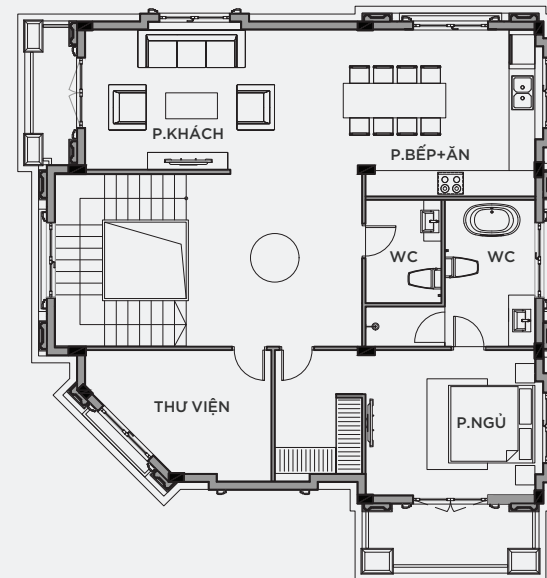
MẶT BẰNG TẦNG 2
