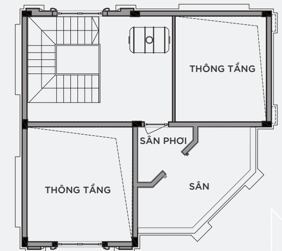
MẶT BẰNG ÁP MÁI
