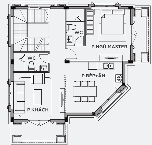
MẶT BẰNG TẦNG 2
