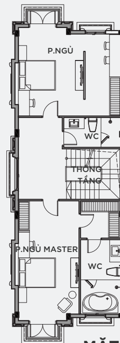
MẶT BẰNG TẦNG 3
