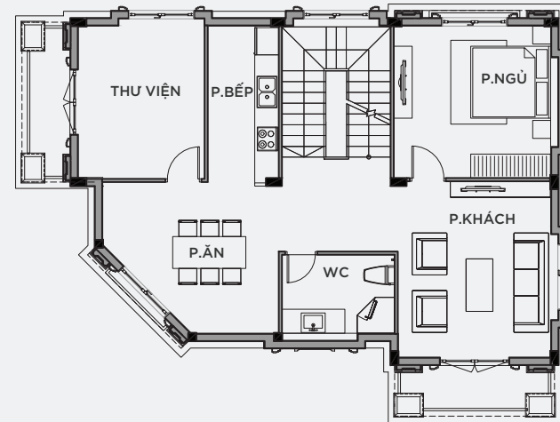
MẶT BẰNG TẦNG 2
