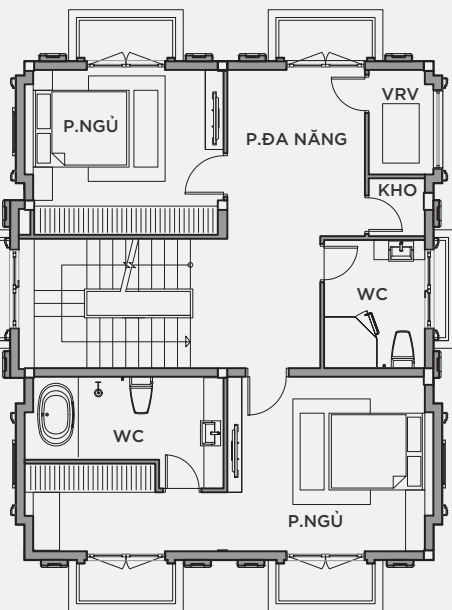
MẶT BẰNG TẦNG 3
