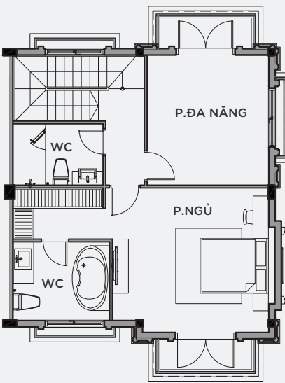
MẶT BẰNG TẦNG 3
