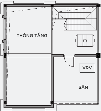
MẶT BẰNG TẦNG TUM
