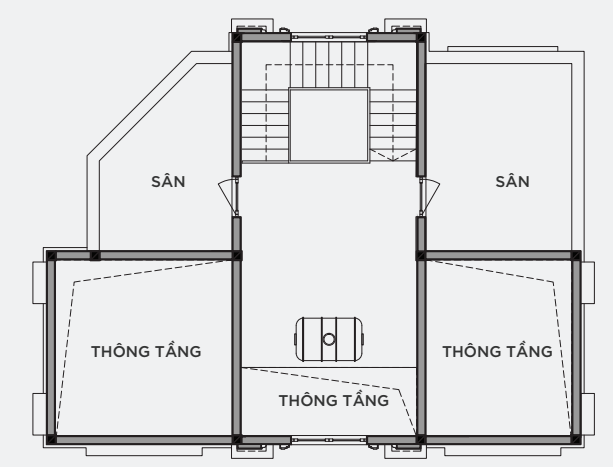
MẶT BẰNG ÁP MÁI
