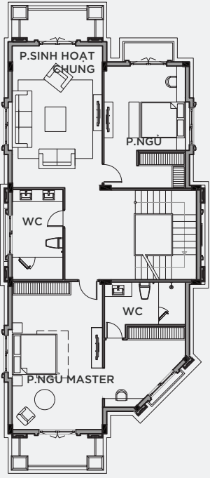
MẶT BẰNG TẦNG 2
