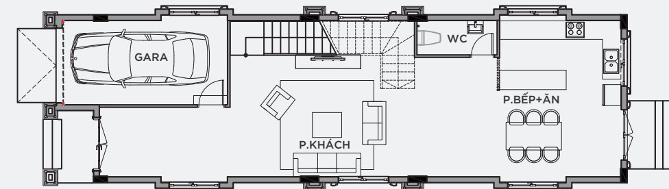
MẶT BẰNG TẦNG 1
