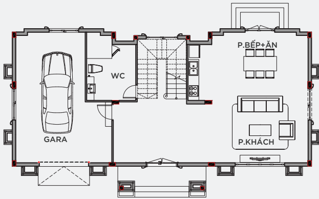
MẶT BẰNG TẦNG 1
