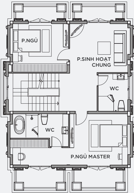
MẶT BẰNG TẦNG 2
