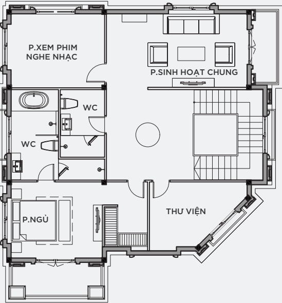
MẶT BẰNG TẦNG 2
