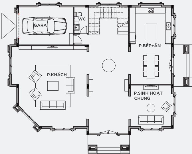
MẶT BẰNG TẦNG 1
