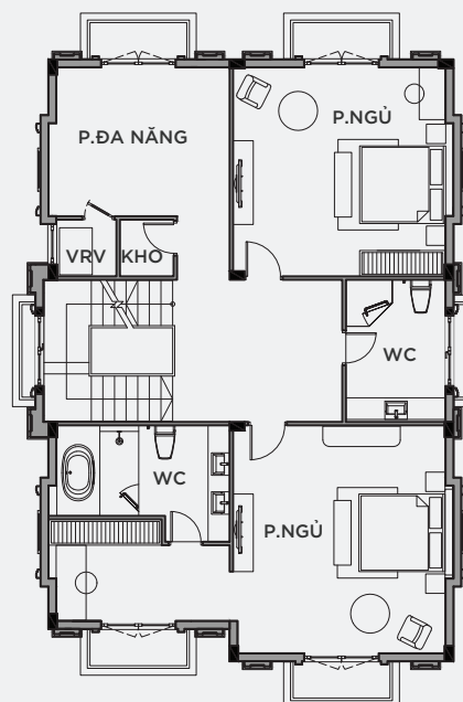
MẶT BẰNG TẦNG 3
