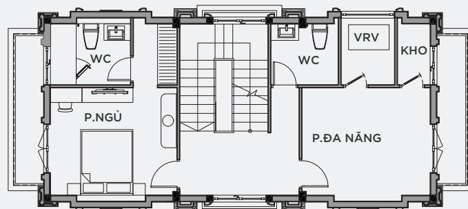
MẶT BẰNG TẦNG 3
