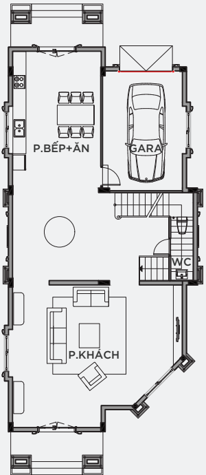
MẶT BẰNG TẦNG 1
