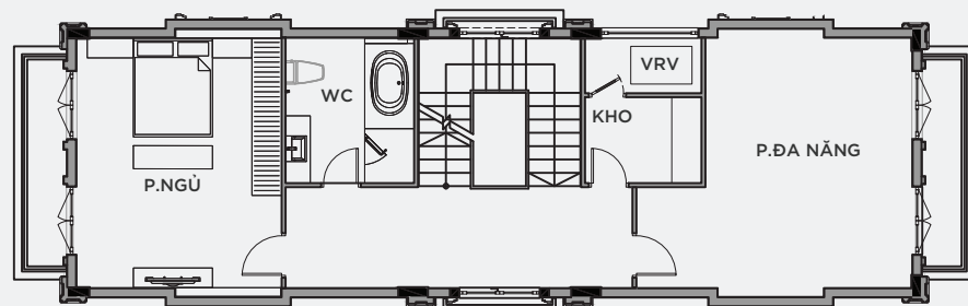
MẶT BẰNG TẦNG 3
