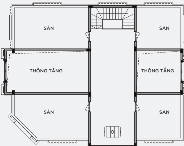
MẶT BẰNG ÁP MÁI
