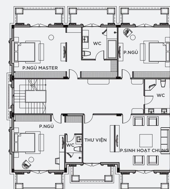
MẶT BẰNG TẦNG 2
