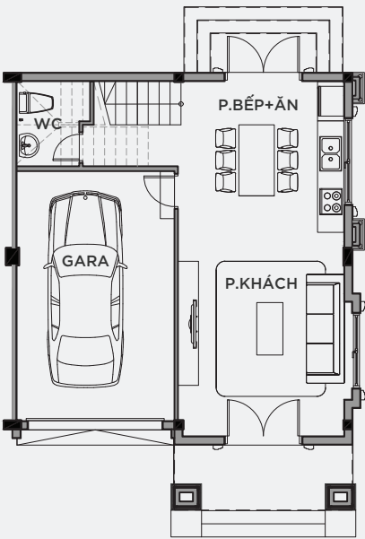
MẶT BẰNG TẦNG 1
