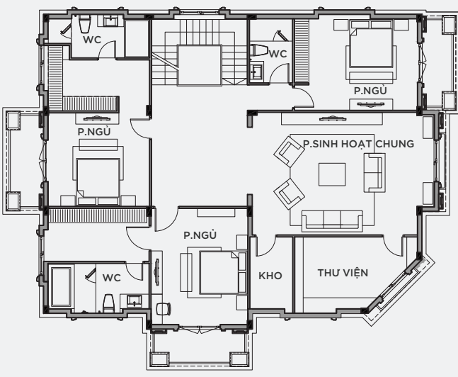
MẶT BẰNG TẦNG 2
