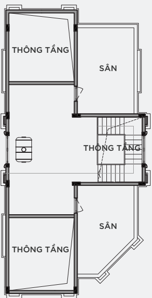
MẶT BẰNG ÁP MÁI
