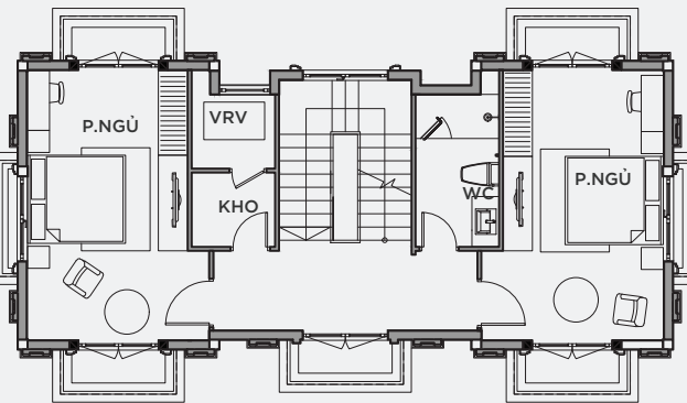
MẶT BẰNG TẦNG 3
