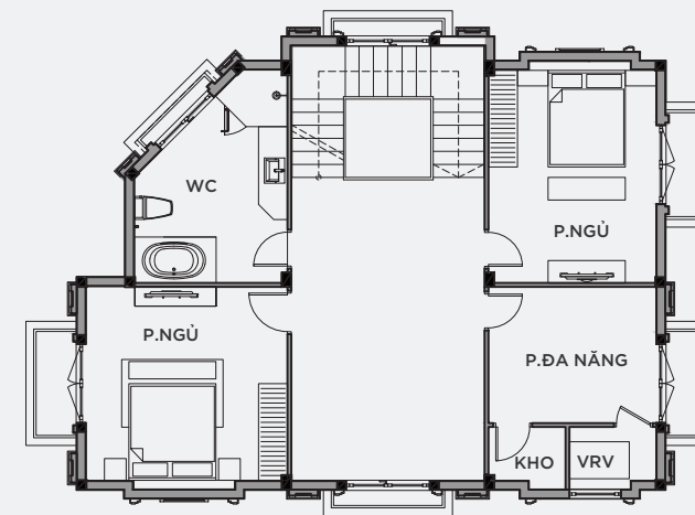
MẶT BẰNG TẦNG 3
