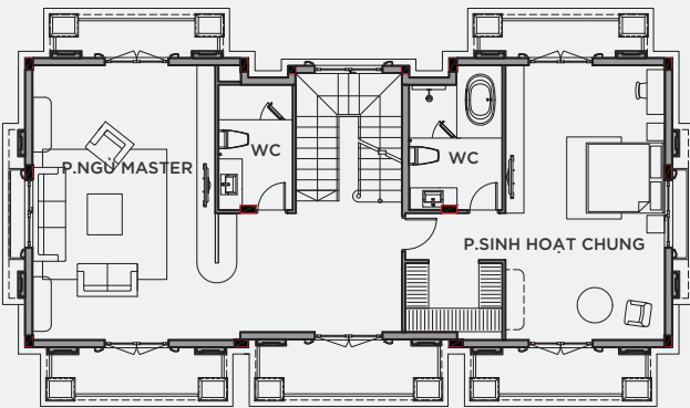
MẶT BẰNG TẦNG 2
