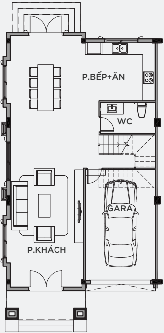
MẶT BẰNG TẦNG 1
