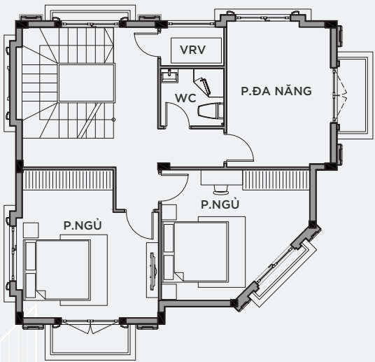
MẶT BẰNG TẦNG 3
