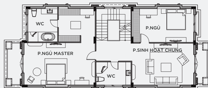
MẶT BẰNG TẦNG 2
