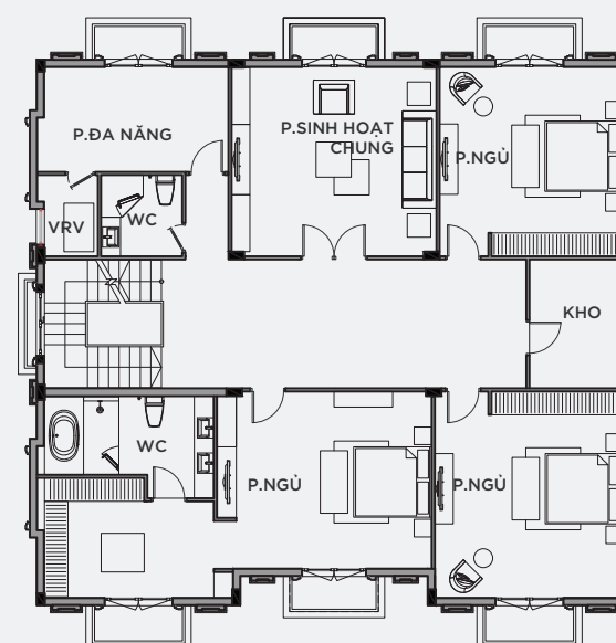
MẶT BẰNG TẦNG 3
