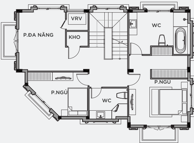
MẶT BẰNG TẦNG 3
