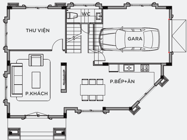
MẶT BẰNG TẦNG 1
