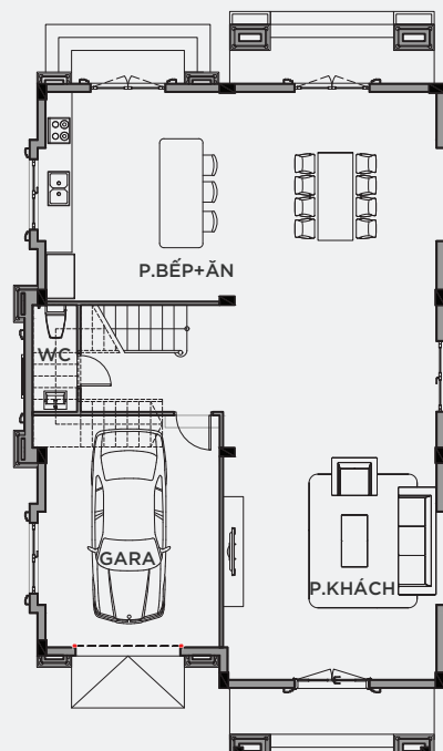
MẶT BẰNG TẦNG 1
