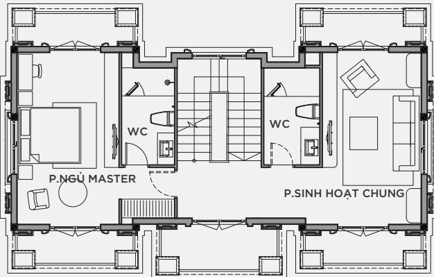
MẶT BẰNG TẦNG 2
