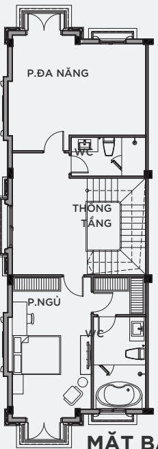
MẶT BẰNG TẦNG 3
