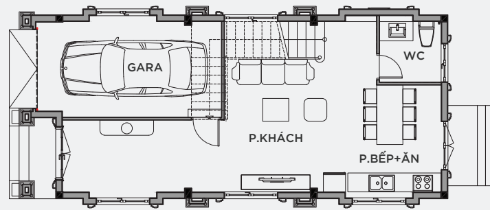
MẶT BẰNG TẦNG 1
