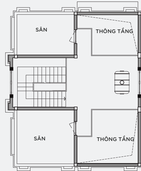
MẶT BẰNG ÁP MÁI
